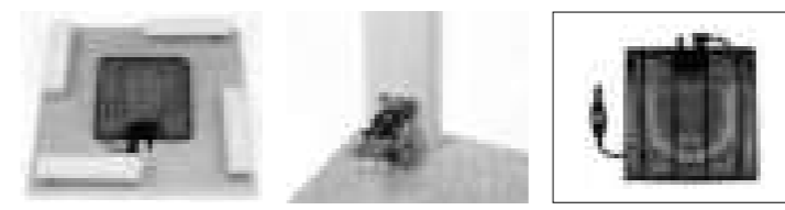
収納に便利な折脚 MS-303H 300W 石英管ヒーター 天板:合成樹脂化粧繊維板(塩化ビニル)/リバーシブル
