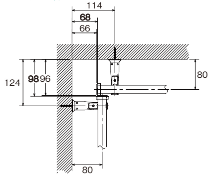
入隅 シングルブラケット付
