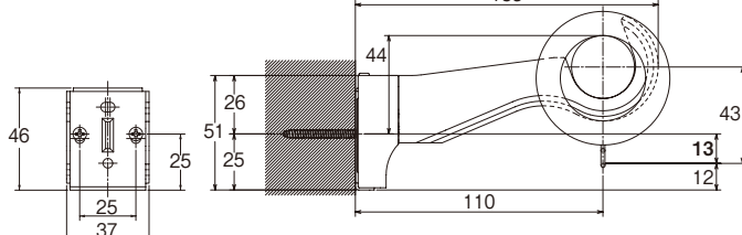
Eダブルブラケット付 (ブラケット幅=50mm)
