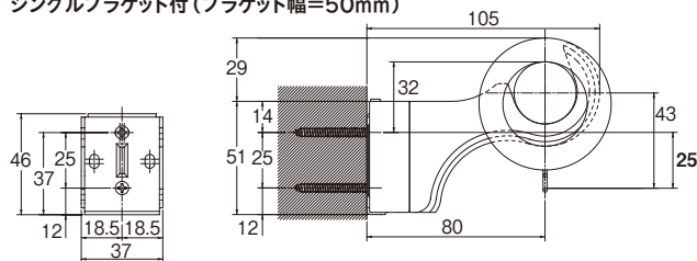
エキストラシングルブラケット付 (ブラケット幅=50mm)
