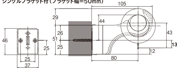
エキストラシングルブラケット付 (ブラケット幅=50mm)
