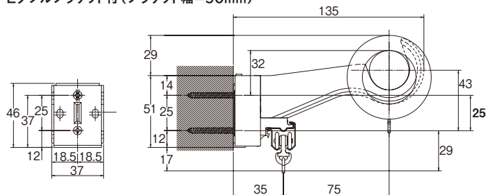
Eダブルブラケット付 (ブラケット幅=50mm)
