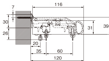
メタルR カバートップIIセット側面図
