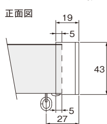
キャップストップMC(ダブル)
