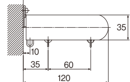
メタルキャップストップM(ダブル) (側面図)
