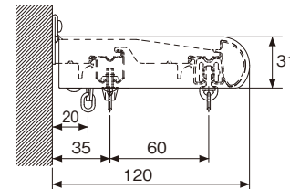
メタルRセット側面図
