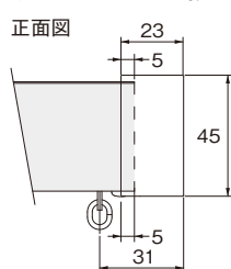
キャップストップMB(ダブル)
