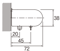
キャップストップ M (シングル) (側面図)
