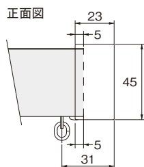
キャップストップMB(シングル)
