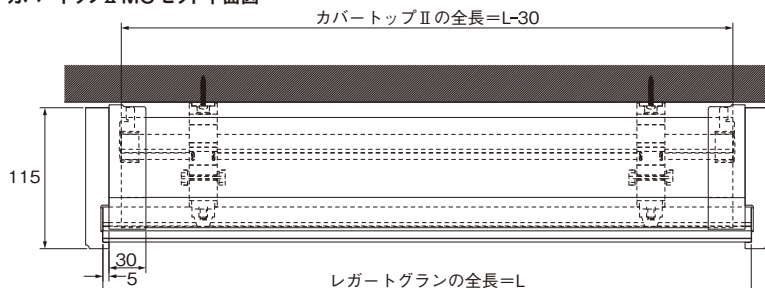
カバートップII MC セット平面図
