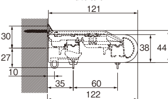
カバートップIIセット側面図
