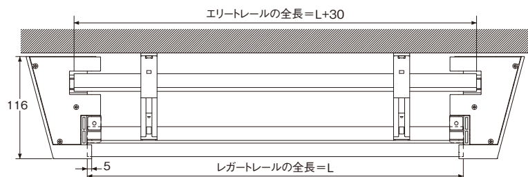
メタルRセット平面図
