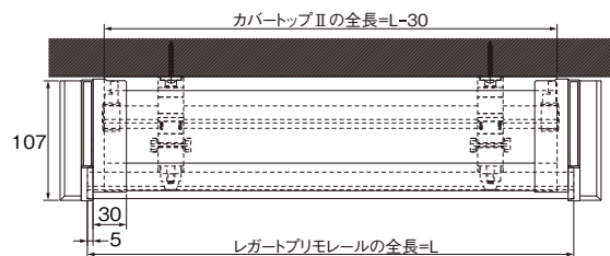
カバートップIIセット平面図
