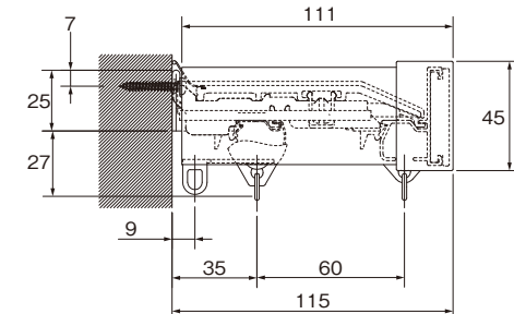
カバートップII MB セット側面図
