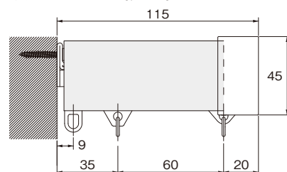
キャップストップMB(ダブル)
