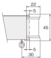
キャップストップA
