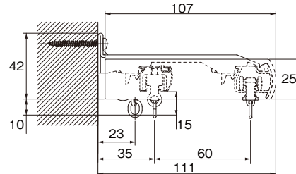
メタルRカバートップIIセット側面図
