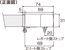
メタルキャップストップR (正面図)
