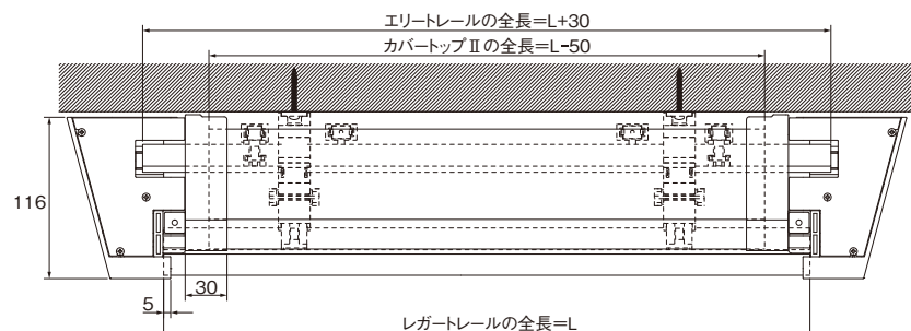
メタルR カバートップIIセット平面図
