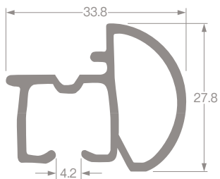
レール断面図 (単位: mm)
