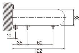
キャップストップ M (ダブル) (側面図)
