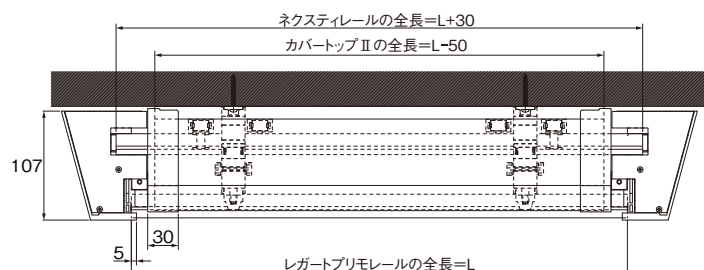
メタルRカバートップIIセット平面図
