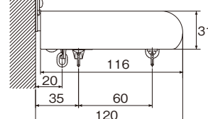
メタルキャップストップR (側面図)
