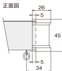
キャップストップMA(シングル)
