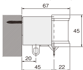
キャップストップMA(シングル)
