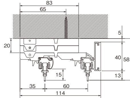
カバートップII MA セット側面図
