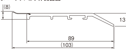
カバートップII本体側面図
