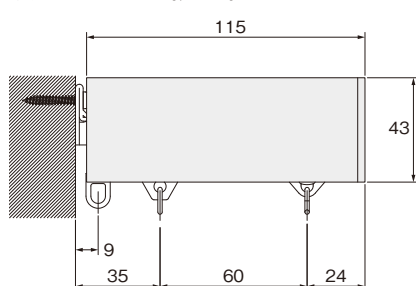
キャップストップMC(ダブル)
