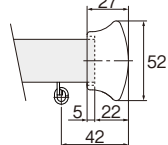
キャップストップM (ダブル)
