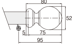
キャップストップM (シングル)
