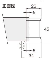
キャップストップMA(ダブル)
