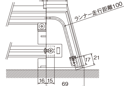
(下面図)
