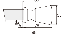
キャップストップ E
