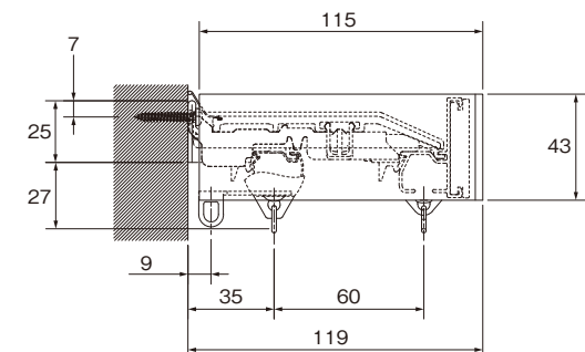
カバートップII MC セット側面図
