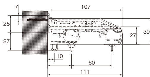
カバートップIIセット側面図
