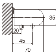
メタルキャップストップM(シングル) (側面図)
