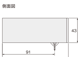
キャップストップMA(ダブル)
