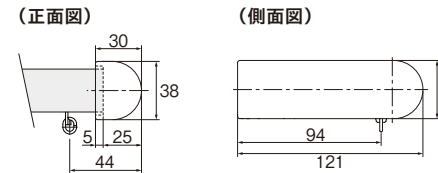
キャップストップM (ダブル)
