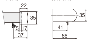
メタルキャップストップM(シングル) (正面図) (側面図)
