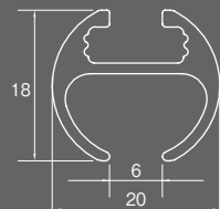
レール断面図 (単位: mm)
