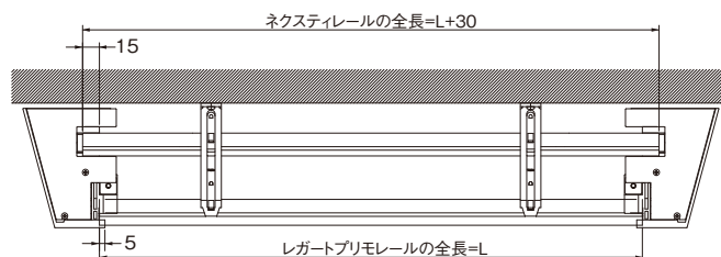
メタルRセット平面図
