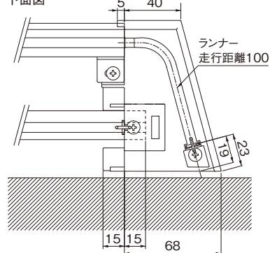
下面図
