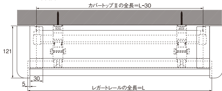
カバートップIIセット平面図
