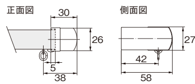
キャップストップM(シングル)
