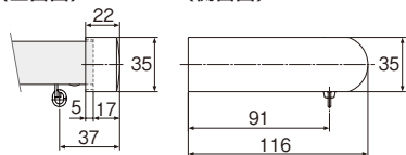
メタルキャップストップM(ダブル) (正面図) (側面図)
