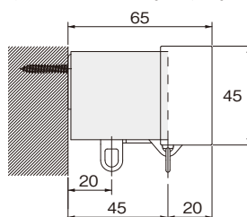
キャップストップMB(シングル)
