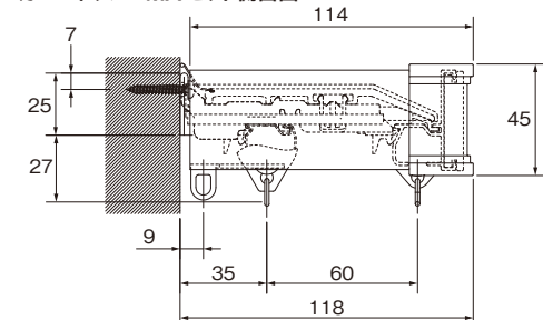
カバートップII MA セット側面図
