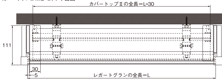
カバートップII MB セット平面図
