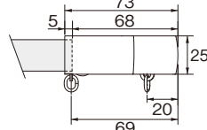
正面図
