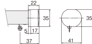
メタルキャップストップ A
