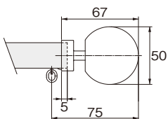
キャップストップM(ダブル)
