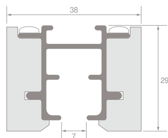
レール断面図 (単位: mm)
