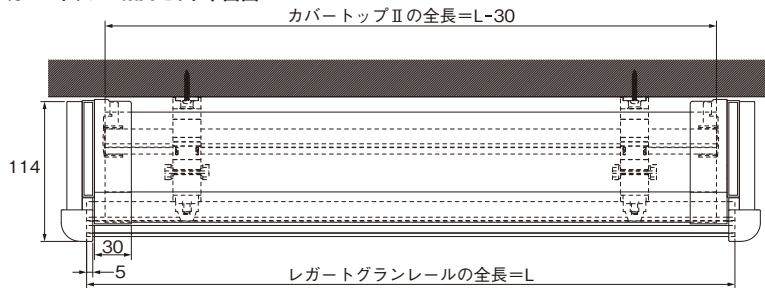
カバートップII MA セット平面図
