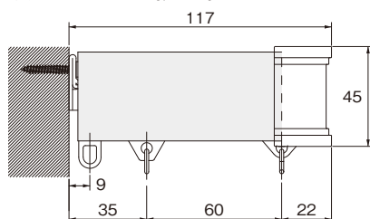
キャップストップMA(ダブル)
