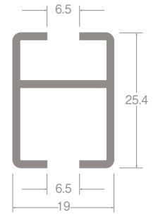
レール断面図 (単位: mm)
