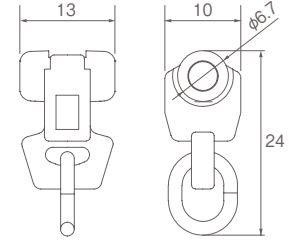
ランナー寸法図 (単位: mm)
