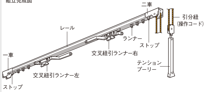
組立完成図
