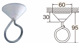
点滴フック寸法図（単位：mm）
