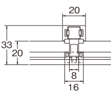
天面図
