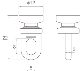
ランナー寸法図 (単位: mm)
