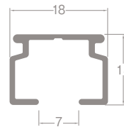
レール断面図 (単位: mm)
