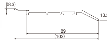
カバートップII本体側面図
