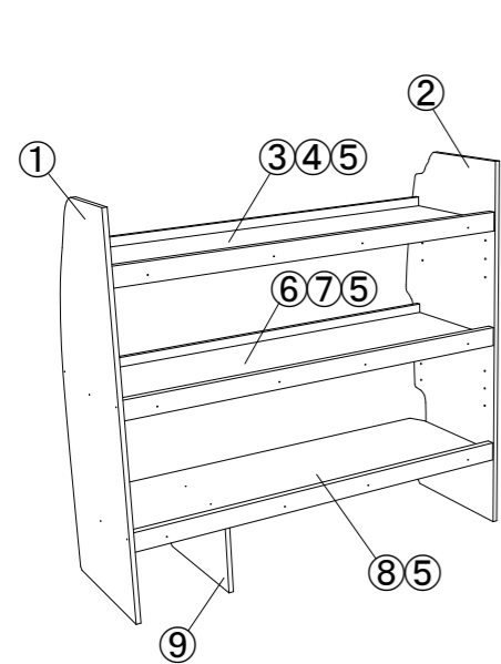
カーゴシェルフ 助手席側用 450mm幅
