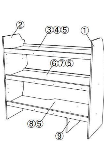
カーゴシェルフ 運転席側用 450mm幅
