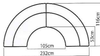
クローネ2個セット時の寸法
