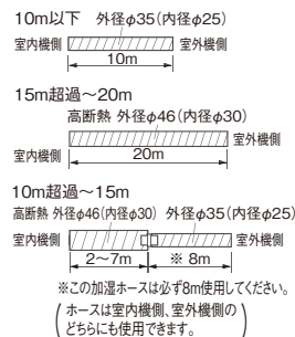
図1: 加湿ホースの必要な長さ
