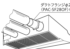
(外気取入用ノックアウト穴(φ200) P80形…2カ所、P140形…3カ所)
