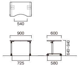
■ラチェット式高さ調節
