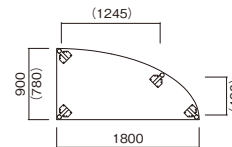
W1800×D900×H700
