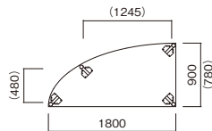
W1800×D900×H700
