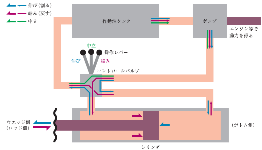
基本な仕組み / 作動油オイルの流れ (MS4000J)
