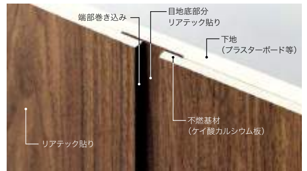
目透かし工法の断面図
