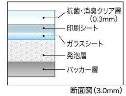
断面図(3.0mm)
