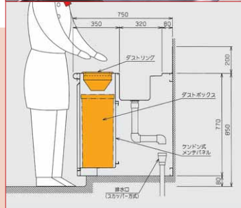
■トラッシュシュート
