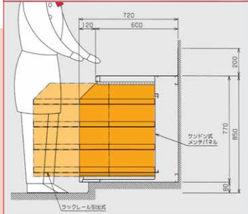
■グラスラック
