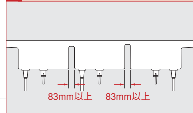
化粧板なしの例
