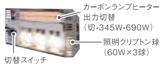
切替スイッチ
