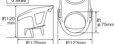
寸法図
