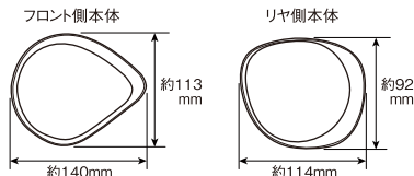
寸法図
