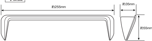
寸法図
