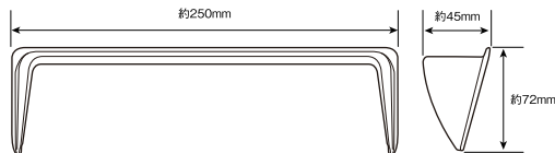
寸法図
